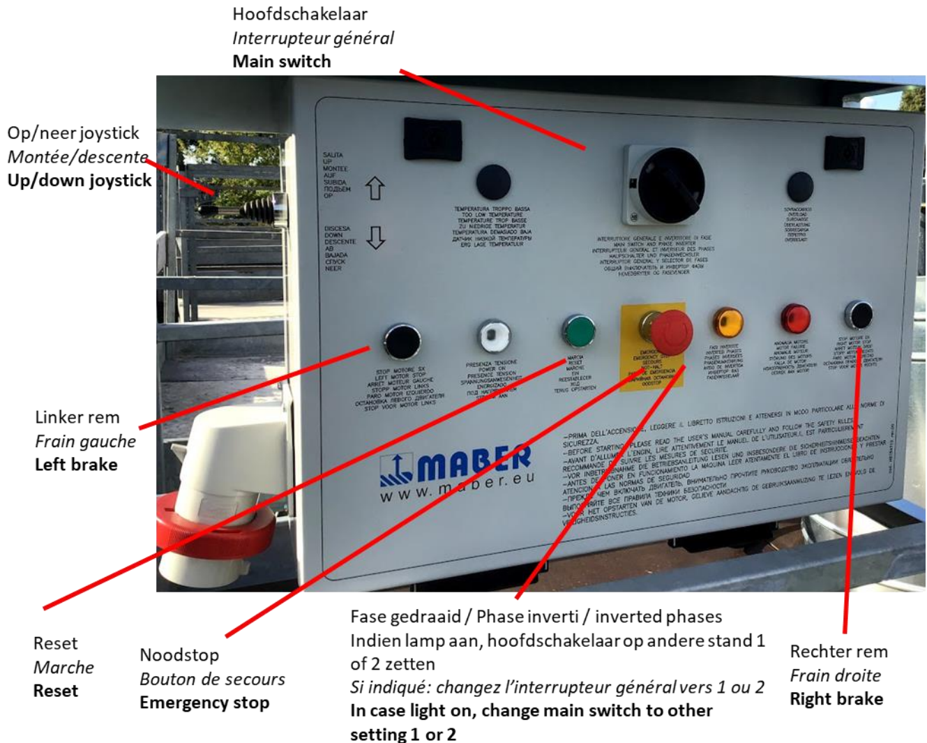
Fig. 1 : Bedieningspaneel op de hefsteiger / Tableau électrique sur la plate-forme de travail / Electrical panel on working platform
